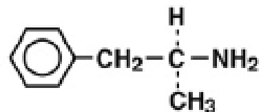
D-Amphetamine
